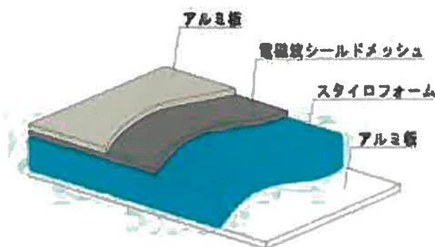
図2. パネル接続は、はめ込み構造により組立工数を削減
